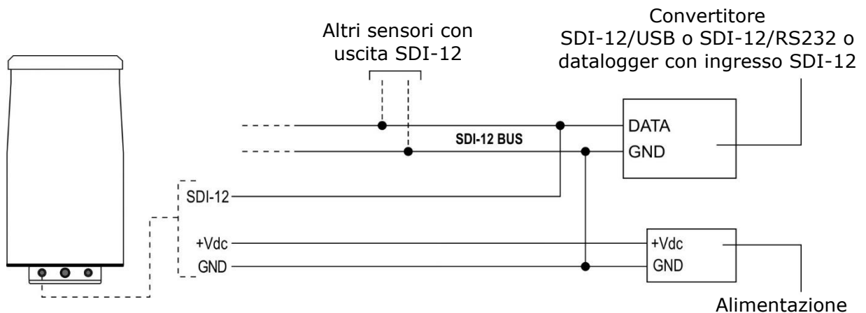
Fig. 4.4.1: collegamento SDI-12
