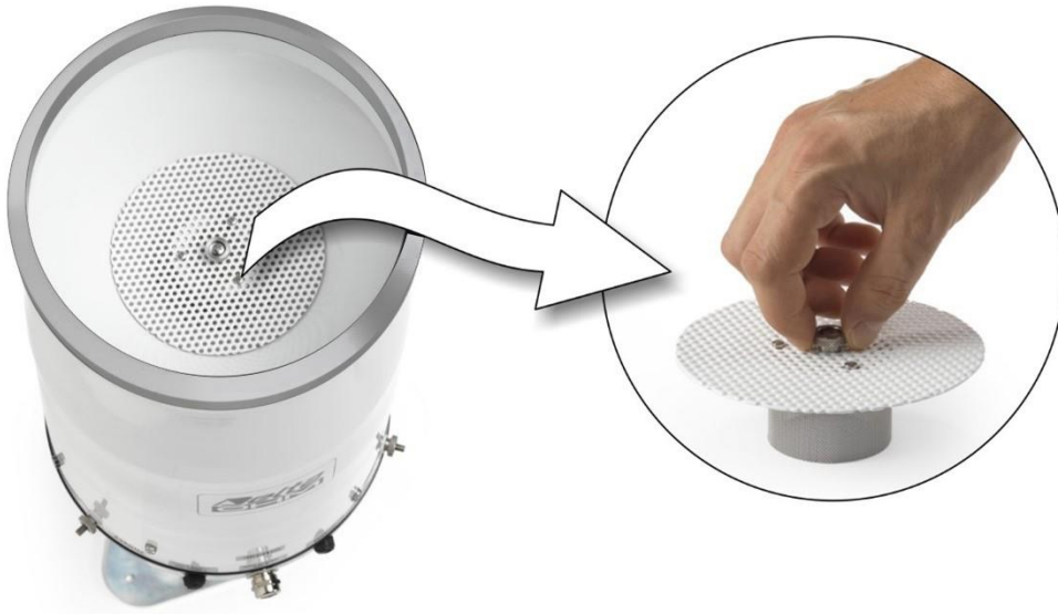
Fig.10.1: filtro superiore
