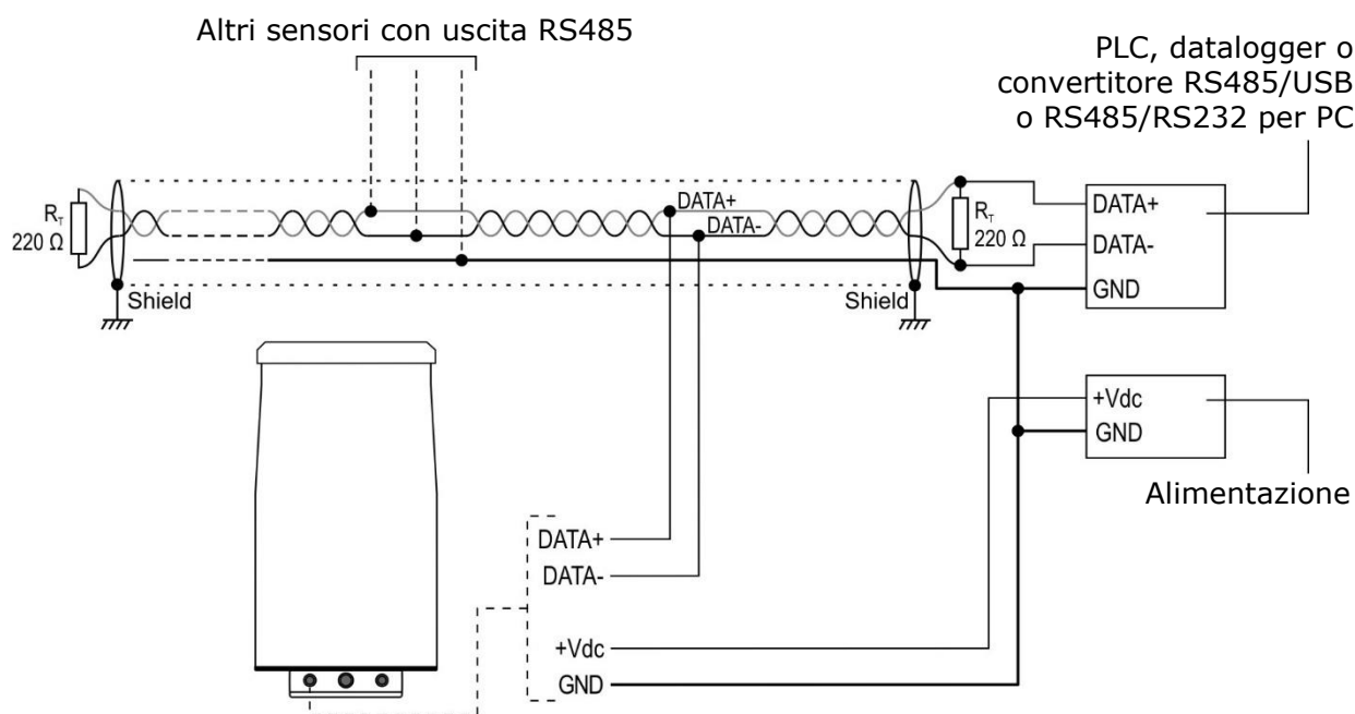
Fig. 4.3.1: connessione RS485
